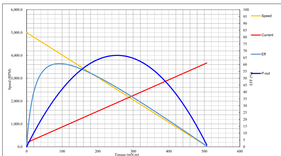
曲线图 Motor Curve
