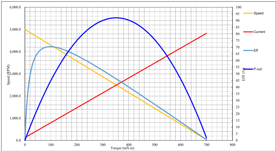
曲线图 Motor Curve
