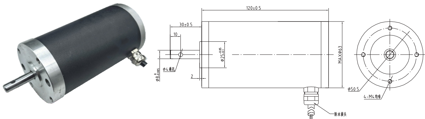
性能参数表 Datasheet
