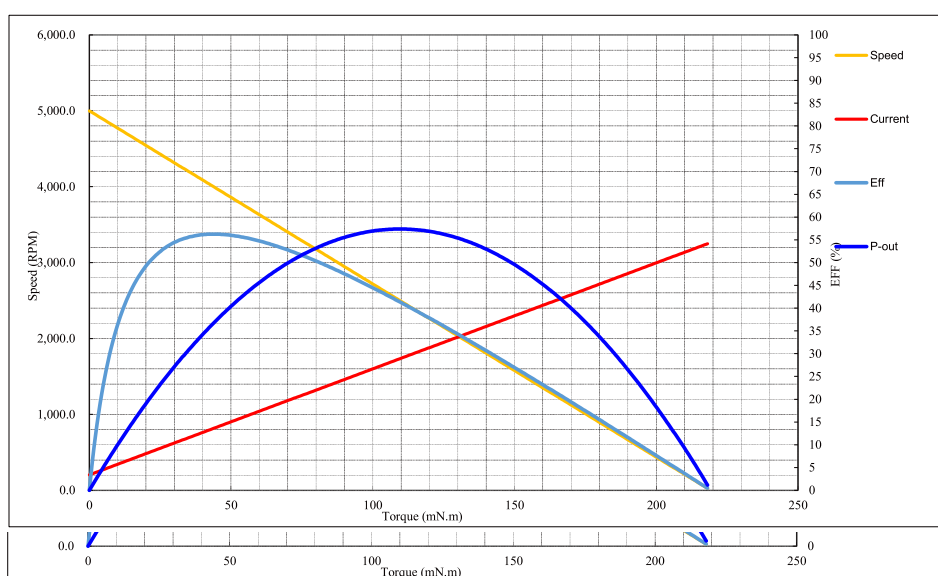
曲线图 Motor Curve
