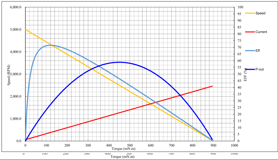
曲线图 Motor Curve
